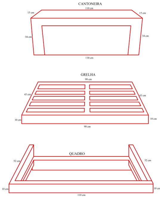
BOCA DE LOBO PADRÃO SUDECAP TIPO "B"
