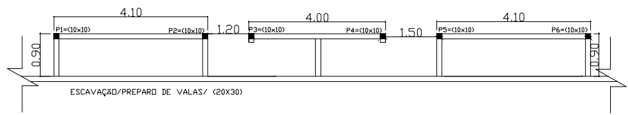
PLANTA BAIXA LOCAÇÃO DOS PILARES 1/100
