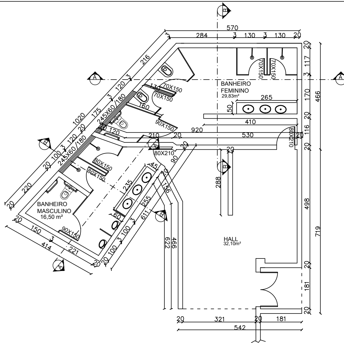
PLANTA BAIXA REFORMA BANHEIROS MASCULINO E FEMININIO ESCALA 1/100
