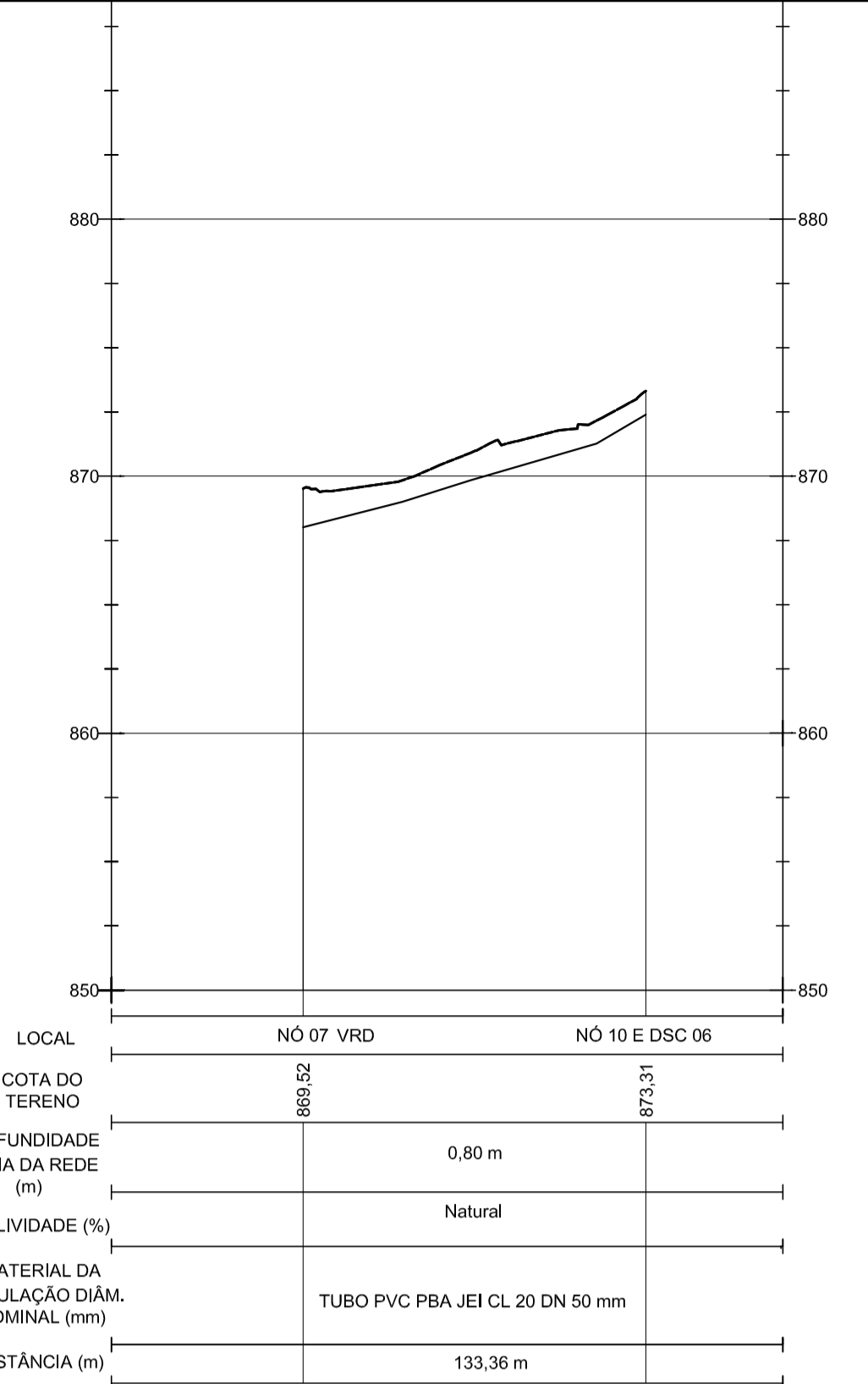
PERFIL LONGITUDINAL DO NÓ 07 AO NÓ 10 ESCALA: H=1:250 V=1:250
