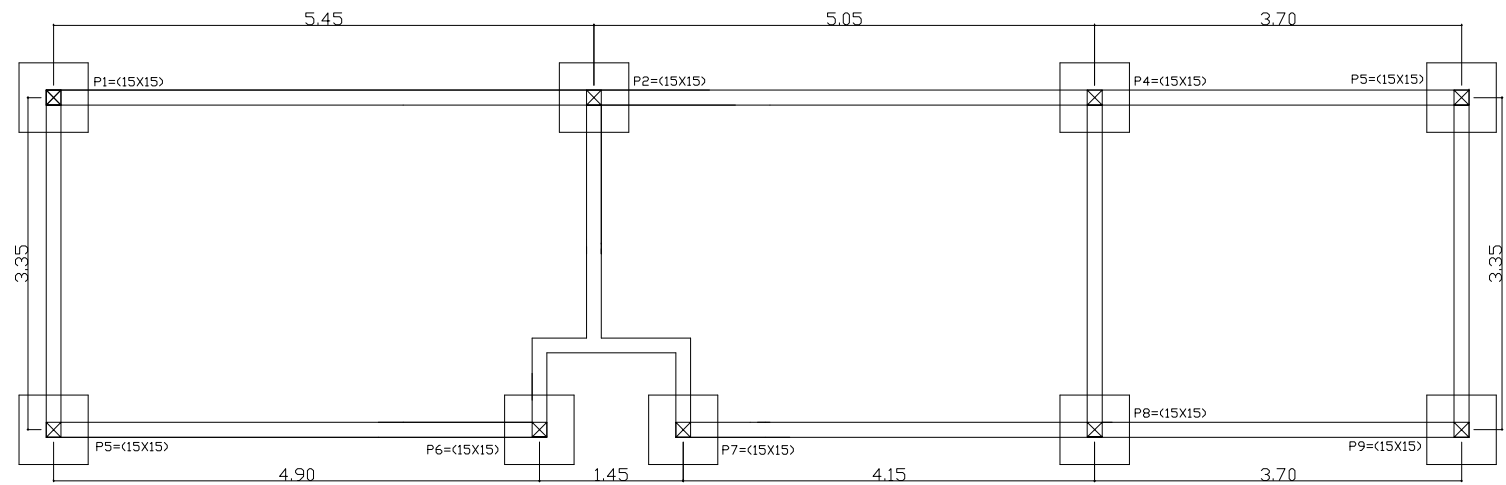
PLANTA BAIXA LOCAÇÃO DOS PILARES 1/50
